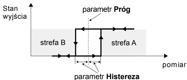
Rys. 7.88. Sterowanie jednoprogowe wyjścia przekaźnikowego
