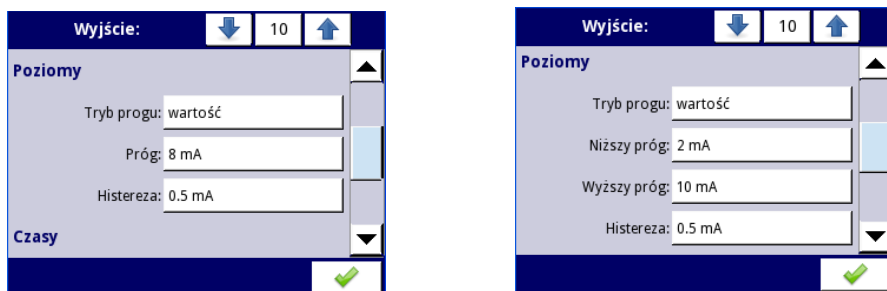
Rys. 7.90. Ustawienia poziomów dla trybu nad progiem i pod progiem (lewy rys.) oraz wewnątrz zakresu i poza zakresem (prawy rys.)
