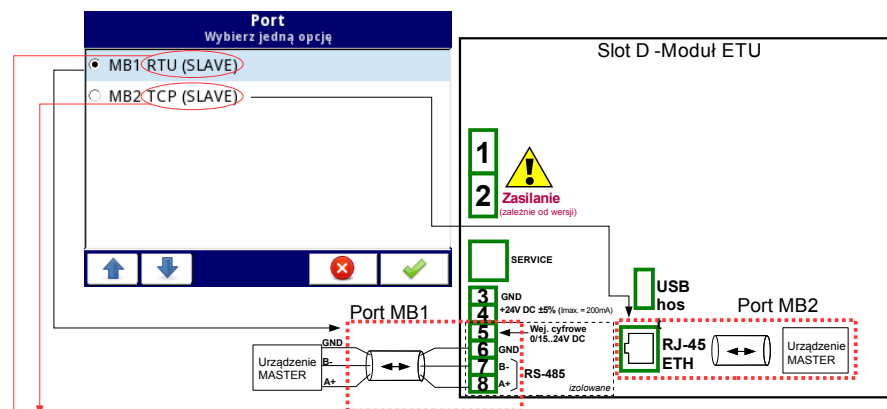
Rys. 7.63. Przykładowe podłączenie urządzenia MultiCon w sieci z podglądem skonfigurowanych portów Modbus
