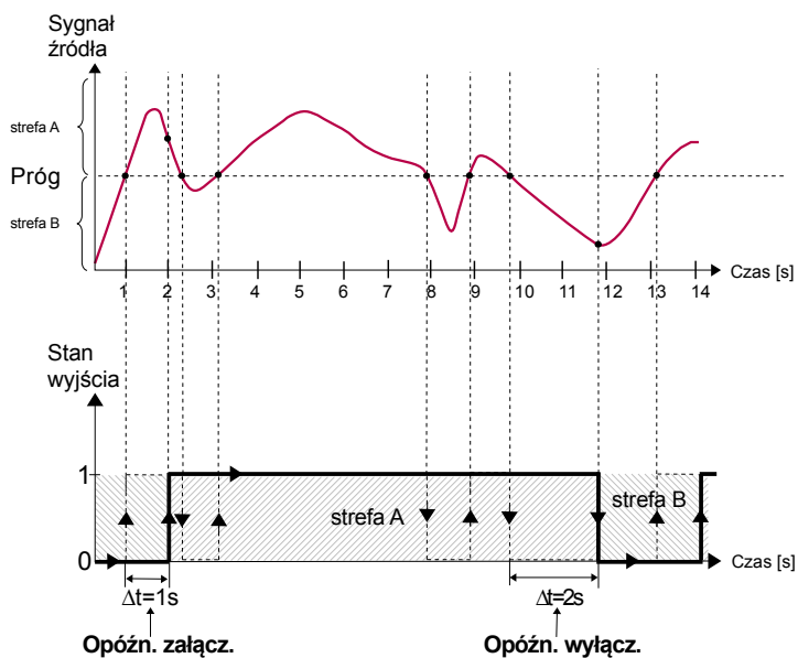
Rys. 7.91. Zasada pracy wyjść przekaźnikowych dla przykładowych ustawień czasowych: Opóźn.załącz. = 1 sec., Opóźn.wyłącz. = 2 sec.
