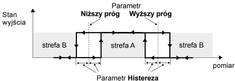
Rys. 7.89. Sterowanie dwuprogowe wyjścia przekaźnikowego
