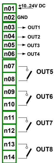
Rys. 8.12. Mieszane moduły wyjść przekaźnikowych
